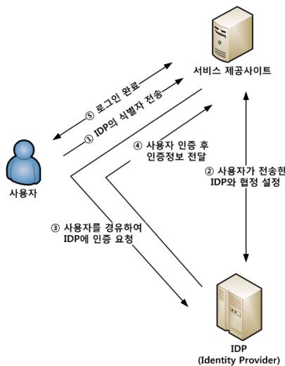
(그림 1) OpenID의 동작방식
