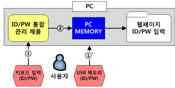
(그림 4) 아이디/패스워드 통합 관리 제품의 동작방식
