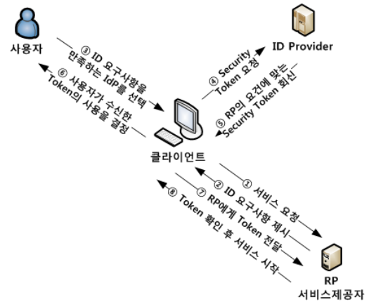
(그림 2) CardSpace의 동작방식
