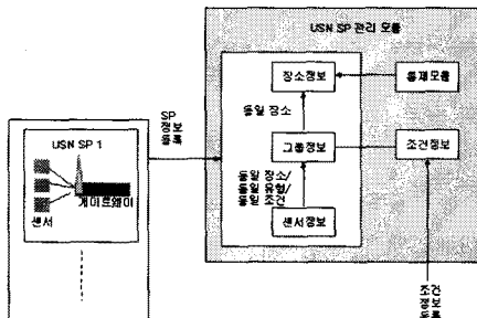
[그림 3] USP SP 정보 관리 모듈
