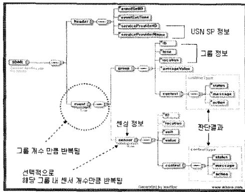
[그림 12] 센서데이터표현언어 구조
