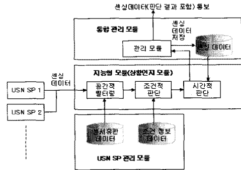
[그림 7] USN 미들웨어의 지능형 모듈
