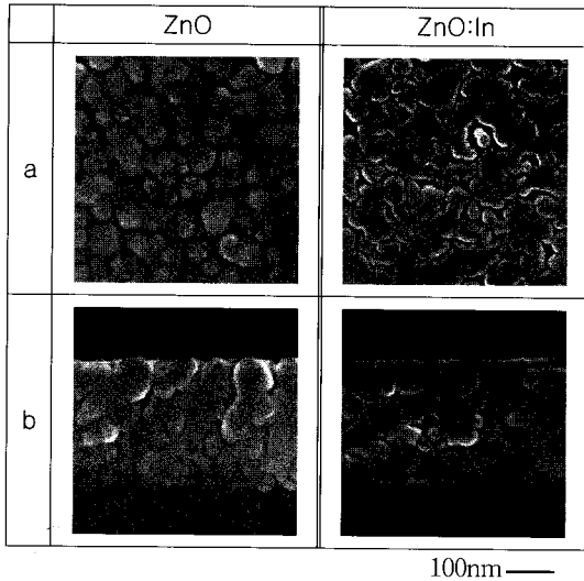
그림 2. 박막의 (a)표면과 (b)단면에 대한 SEM 사진.
