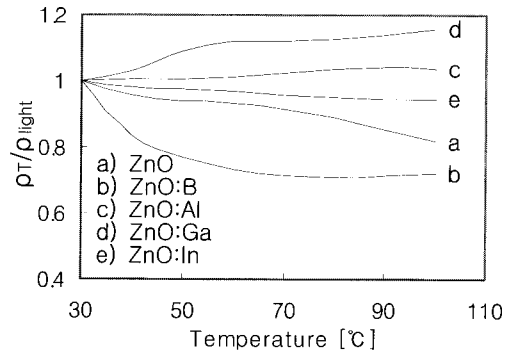
그림 7. 광저항의 온도의존성.
