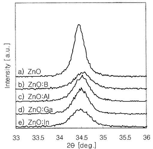
그림 1. 박막의 XRD 곡선.
