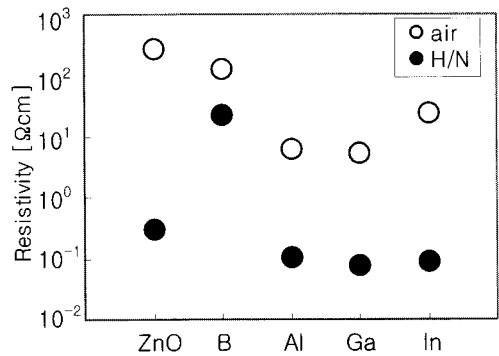
그림 5. 도핑물질에 대한 저항률(O:공기중에서 1차 열처리, ●:수소/질소 분위기에서 2차 열처리).
