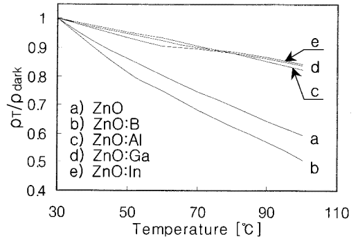
그림 6. 암저항의 온도의존성.
