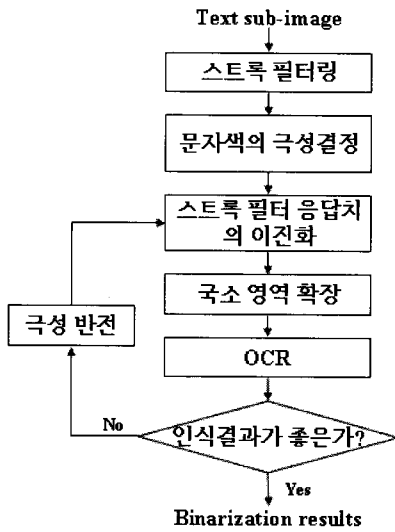
그림 4. 알고리즘의 흐름도
