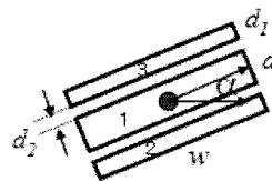
그림 5. 스트록 필터
