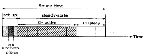
그림 4. 제안 방식의 라운드 구조 Fig. 4 Round format of proposed scheme
