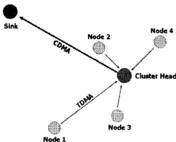
그림 1. LEACH 프로토콜의 클러스터 구조 Fig. 1 Cluster structure of LEACH protocol
