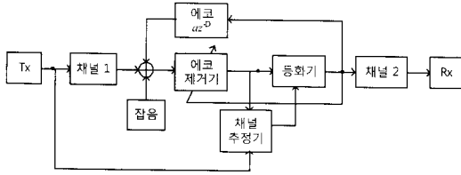
그림 3. 등화기반 TD-MB 중계기 시스템 구조
