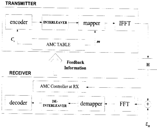
그림 1. 적응변조 BIC-OFDM 시스템 Fig. 1 System model for the adaptive BIC-OFDM
