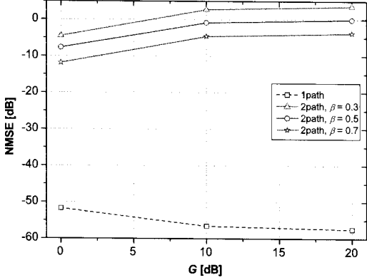
그림 4. 경로별 채널 추정 시 추정값 \hat{\alpha}_0 의 NMSE (중계기 SNR = 30 dB)
