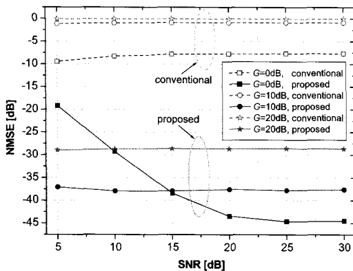
그림 5. \beta = 0.5 인 경우 중계기 SNR의 변화에 따른 NMSE
