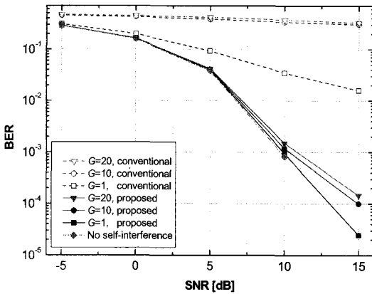
그림 7. 중계기 신호를 수신하는 단말기 BER 성능( \beta = 0.5 , 중계기와 단말기 사이의 채널 환경: AWGN)
