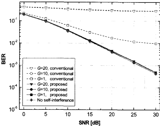
그림 8. 중계기 신호를 수신하는 단말기 BER 성능 ( \beta = 0.5 , 중계기와 단말기 사이의 채널 환경: Vehicular-A 채널, 단말기 이동속도 30 km/h)
