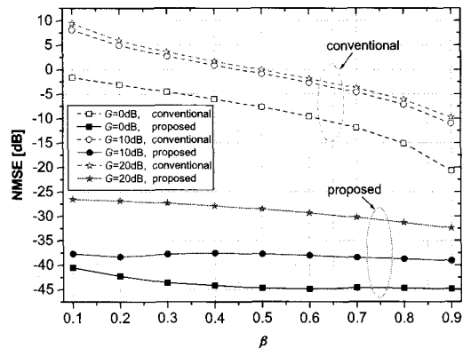
그림 6. \beta 의 변화에 따른 추정 방식별 \hat{\alpha}_0 의 NMSE (중계기 SNR = 30 dB)
