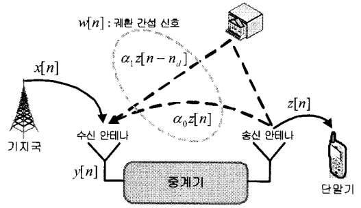
그림 1. 다중 궤환 간섭 신호를 갖는 중계기 모델
