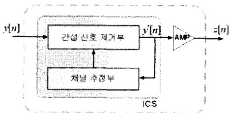
그림 2. 채널 추정부와 간섭 신호 제거부를 포함하는 ICS 중계기 구조
