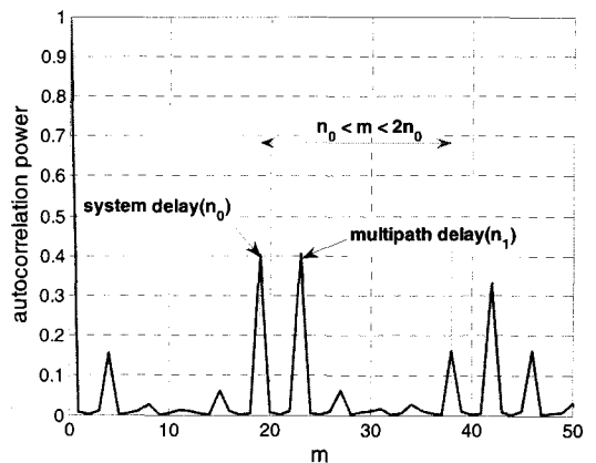
그림 3. 수신 신호 y[n] 의 자기 상관 함수
