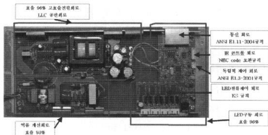
그림 4. 시제품의 외형 Fig 4. Cofiguration of LED System
