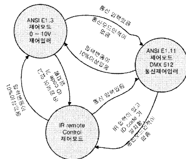
그림 3. 사용자 입력에 따른 조명단말기의 제어 Fig 3. Control of LED Terminal for the User's Input
