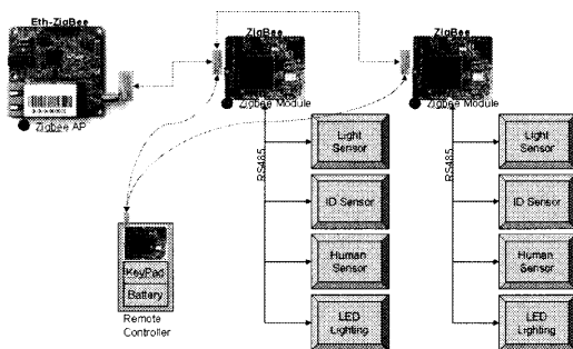
그림 2. 무선으로 구성된 지능형 조명 제어 시스템 Fig 2. Intelligent LED System Using the Wireless Control
