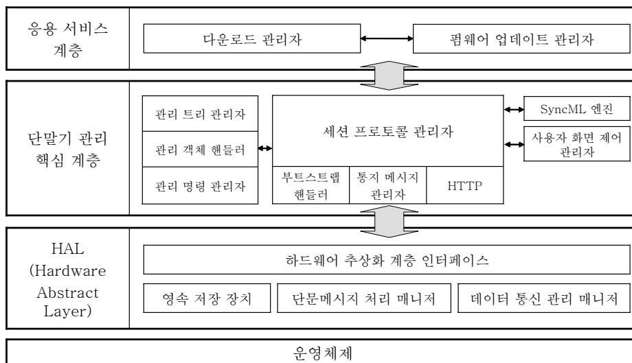
(그림 2) 각 계층별 MDM 에이전트의 세부 구조
