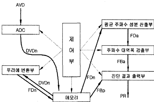
그림 3. 진단기기의 구성도
