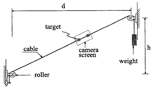
Fig. 3 Test setup
