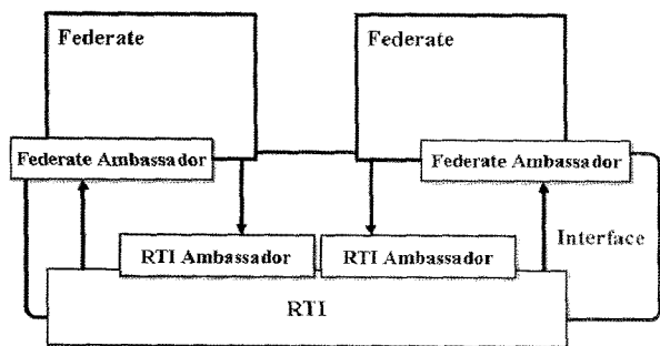
그림 5 HLA/RTI Structure
