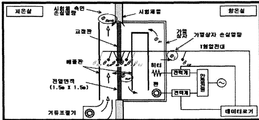
[그림 2] 열관류율 시험방법 및 손실열량의 표현
