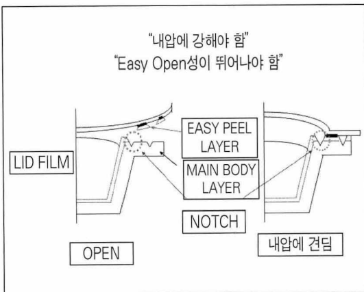
[그림 2] MAGIC TOP 용기 기본구조
