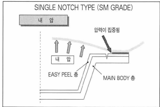
[그림 7] 강한 내압(밀봉성) 원리
