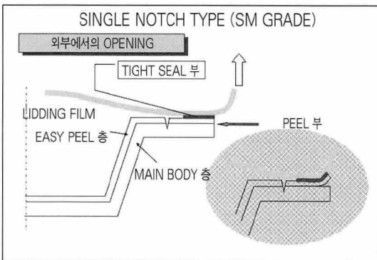
[그림 6] 리드필름 이지필 원리
