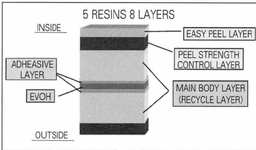
[그림 5] MAGIC TOP 시트 구조
