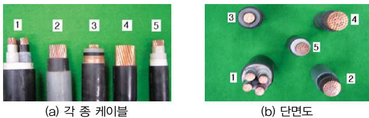
사진 5. 각 종 케이블과 단면도
