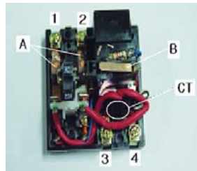
사진 2. 누전차단기 내부
