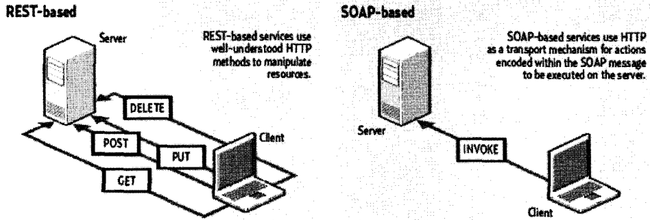
<그림 8> 검색 기법: REST vs SOAP 22)
