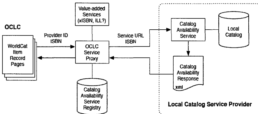
<그림 10> Catalog Availability Web Services: Architecture
