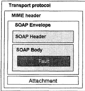
<그림 5> SOAP 기본 구조
