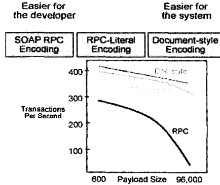
<그림 6> SOAP 인코딩 스타일
