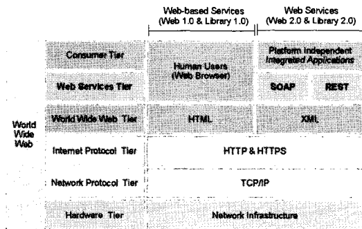
<그림 4> 웹서비스 스택 17)
