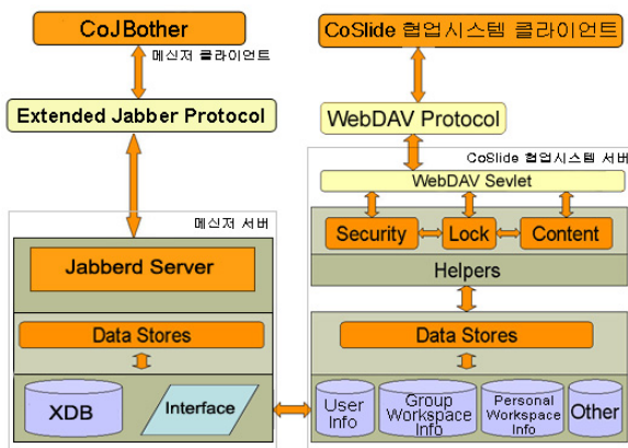
(그림 5) 협업시스템의 구조와 함께 연동된 메신저 시스템의 구조
