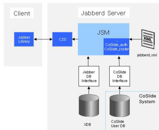
(그림 11) 협업시스템과 연동한 Jabber Server의 구조
