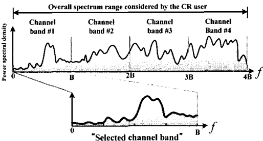
그림 3. 스펙트럼 유희도 인지를 통한 최적의 채널 대역 선택에 대한 예.
