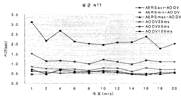
(그림 8) 평균 NET_TRAVERSAL_TIME
