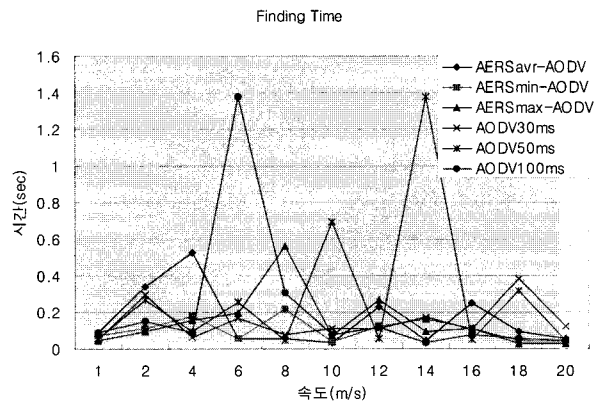
(그림 7) 소스 노드에서 목적지 노드까지 메시지 전송 소요시간
