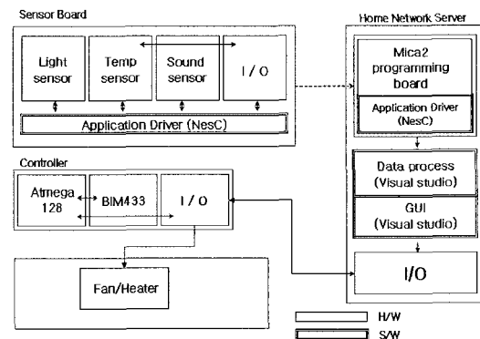
그림 18. 실내 온도 자동 조절기 구조도 Fig. 18. Structure of automatic temperature controller
