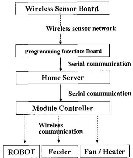
그림 4. 애완견 관리용 무선 지능 시스템 전체 구조도 Fig. 4. Overall structure of pet management system
