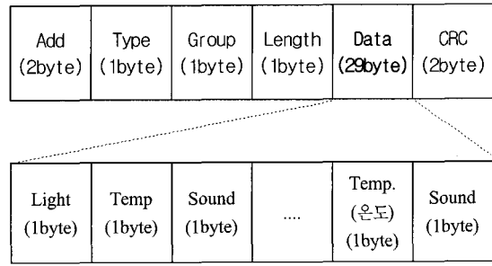
그림 7. 프로토콜(36바이트) 및 데이터 프레임 구성 Fig. 7. Protocol and data frame
