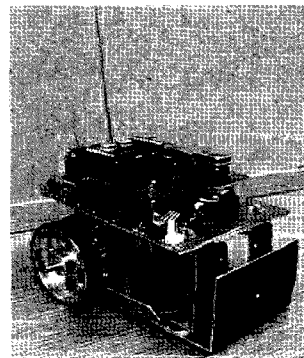
그림 13. 애완견 유도용 미니로봇 시스템 Fig. 13. Mini-robot system for pet guidance
