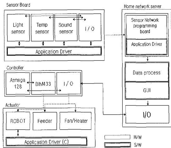
그림 10. 전체 시스템 구성도 및 동작 개요 Fig. 10. Overall System Structure
