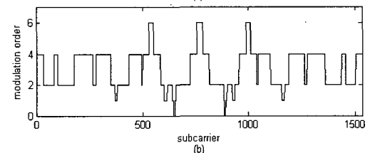
그림 3. 적응전송 SISO-OFDM 시스템에서 채널 값에 따른 변조방식 결정 (a) 각반송파의 채널 값과 문턱값 (b) 각 부반송파의 채널 값에 따른 변조지수
