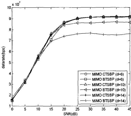
그림 13. MIMO-OFDM 시스템에서의 CTSBP와 BTSBP의 데이터 율 비교 (CESNR 50dB)
