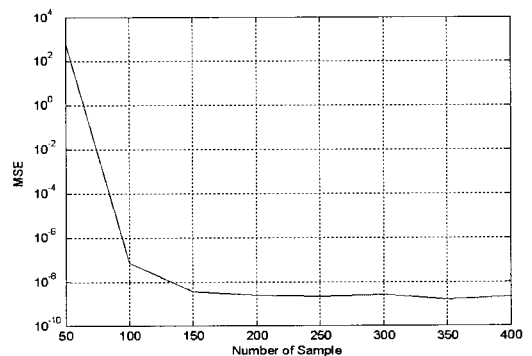
그림 8. 채널 예측 필터의 기중치벡터 생성에 사용되는 샘플 수에 따른 MSE
