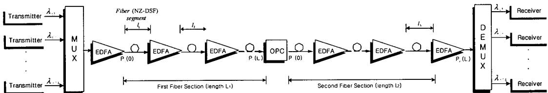
그림 1. 24 채널 x 40 Gbps WDM 시스템
