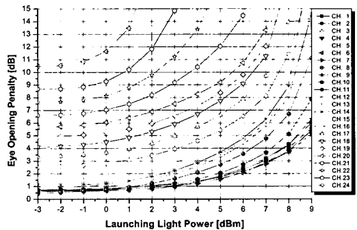
그림 5. MSSI 기술이 적용된 WDM 시스템에서 입사 전력에 따른 EOP
