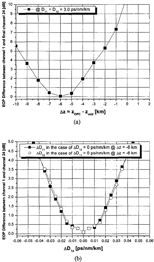
그림 6. 채널 1과 24의 EOP 차이. (a) D_{11} = D_{12} = 3 ps/nm/km에서 \Delta z 에 의존하는 경우, (b) 그림 (a)에서 구한 최상 \Delta z 에 OPC가 위치하고 \Delta D_{1x} 에 의존하는 경우
