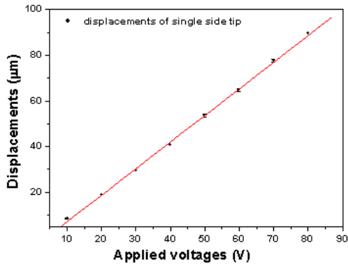
그림 16. In-plane 압전형 마이크로 그리퍼의 입력 전압과 변위의 관계
