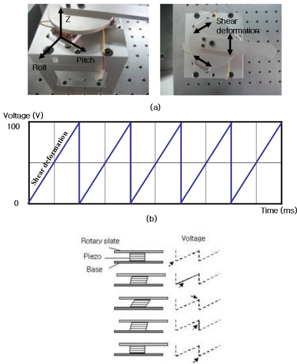
그림 4. 전단변형 압전소자 기반 회전 메커니즘, R-type 1
