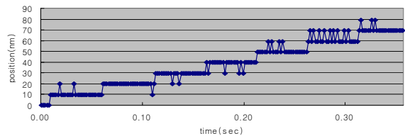
그림 14. 선형 P-type 1의 분해능
