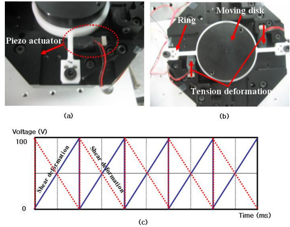
그림 5. 인장변형 piezo actuator기반 회전 메커니즘
