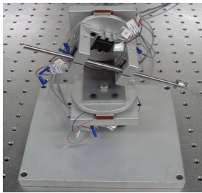
그림 7. R-R-P형 매니플레이터
