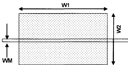
그림 3. 사각형 DGS를 지닌 마이크로스트립 선로 Fig. 3. Microstrip line with rectangular DGS.
