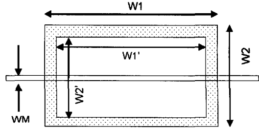
그림 4. 사각형 DGS와 아일랜드를 지닌 마이크로스트립 선로
