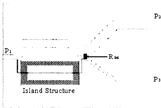
그림 6. 가변 윌킨슨 전력 분배기의 PCB 레이아웃 Fig. 6. PCB layout of the variable unequal Wilkinson power divider.
