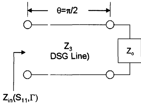
그림 2. DGS 선로의 특성 임피던스를 구하기 위한 등가 모델
