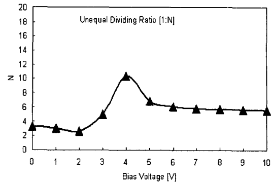
그림 9. 바이어스 전압에 따른 1:N 비대칭 분배 비율의 측정 결과
