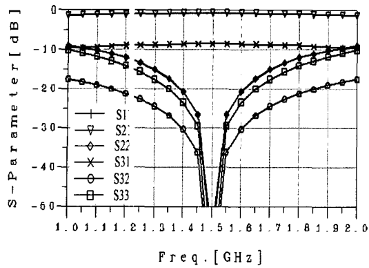
(a) 이상적인 전송 선로로 구성된 경우 (a) Circuit simulation using ideal elements
