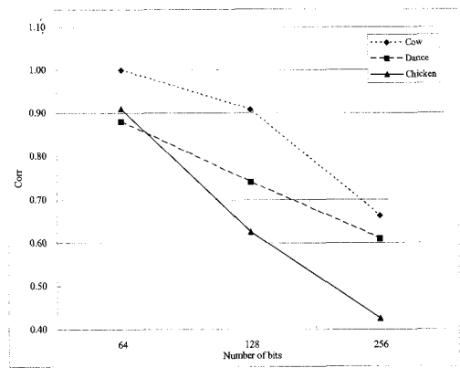
그림 9. 삽입강도를 고정( \Delta = 0.08 )하고 삽입 비트수를 달리하여 워터마크를 삽입 한 후 균일 양자화 공격을 가한 후 워터마크 검출 결과
