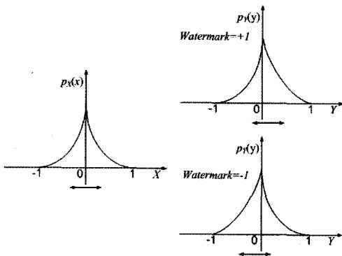
그림 4. 워터마크 비트에 따른 라플라시안 분포의 비대칭적 수정 Fig. 4. Asymmetric modification of Laplacian distribution according to the watermark bit
