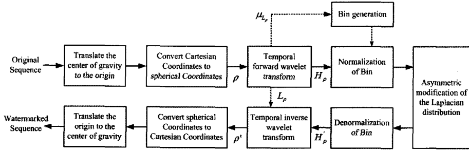
그림 3. 워터마크 삽입 과정 Fig. 3. Block diagram of the watermark embedding procedures
