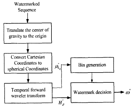
그림 5. 워터마크 검출 과정 Fig. 5. Block diagram of the watermark extraction procedures
