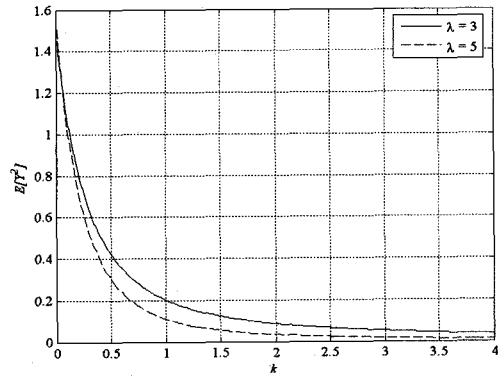
그림 A-1. 입력 랜덤 변수가 라플라시안 분포를 가질 때, 히스토그램 대응 함수의 파라미터 k 값에 따른 출력 변수의 2차 모멘트
