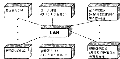
(그림 3) 개선된 하나로 RMS 컴퓨터 연결도
