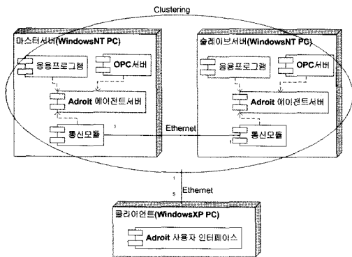
(그림 13) RMS 소프트웨어 아키텍처
