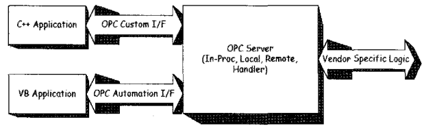
(그림 10) OPC 인터페이스 개념도
