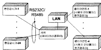
(그림 2) 기존의 하나로 RMS 컴퓨터 연결도
