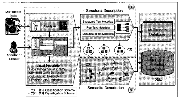
(그림 11) SMAT 전체적인 작업흐름
