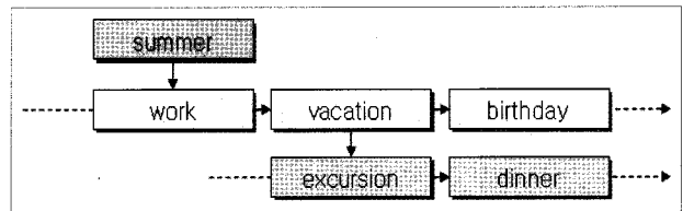
(그림 3) “summer” 예시 멀티미디어 데이터 구조
