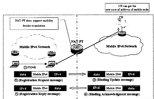
그림 13. Mobile IPv4 노드와 IPv6 간 등록과정
