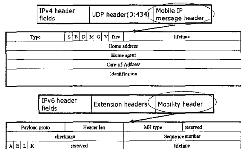
그림 10. Mobile IPv4 헤더와 Mobile IPv6 헤더
