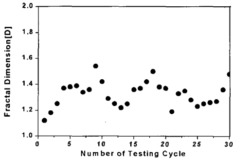
그림 4. EPDM 애자의 가속실험 결과 (저비중). Fig. 4. Result of acceleration in EPDM-1.
