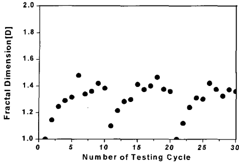
그림 3. 실리콘 애자의 가속실험 결과. Fig. 3. Result of acceleration in silicone insulators.
