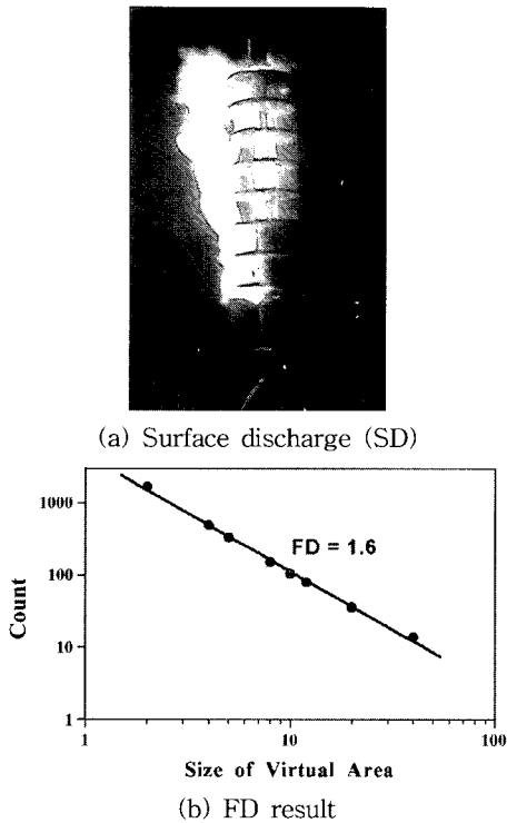
그림 1. 가속 사이클 후에 발전된 표면방전(SD) 및 프랙탈 차원 (FD). Fig. 1. Surface discharge (SD) and fractal dimension (FD) after acceleration.
