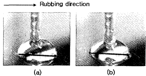
그림 4. 러빙 처리한 기판 위에서의 전압 인가에 따른 탈이온수의 접촉각 변화: (a) 전압 인가 전 및 (b) 전압 인가 후. Fig. 4. Contact angle variation of deionized water on substrate which has rubbing treatment: (a) before and (b) after the applied voltage.
