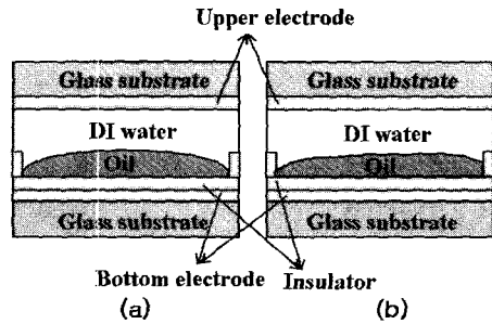
그림 2. 탈이온수와 오일의 접촉 단면도: (a) 이상적인 경우 및 (b) 실제 경우.
