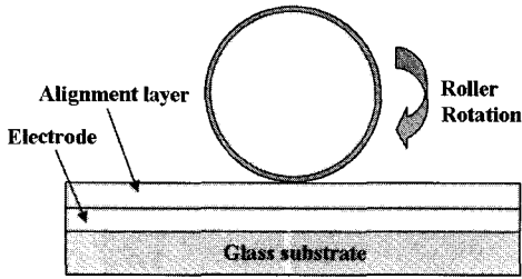
그림 3. 배향막 표면 처리를 러빙 방법. Fig. 3. Rubbing method for surface treatment of alignment layer.
