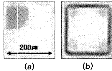
그림 8. 부분 식각된 전극을 사용한 단위셀의 구조: (a) 한 구석이 부분 식각된 전극 과 (b) 네 구석이 부분 식각된 전극. Fig. 8. Operation of EWD test cells using patterned electrode: (a) partial etched electrode at one corner, and (b) partial etched electrode at four corners.
