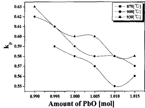
그림 4. PbO량에 따른 전기기계결합계수 k_p . Fig. 4. Electromechanical coupling factor k_p with the amount of PbO.
