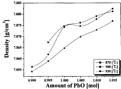
그림 1. PbO량에 따른 밀도.
