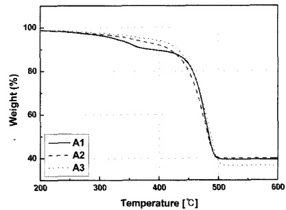
(b) 현재 사용 중인 반도체 재료의 TGA curve
