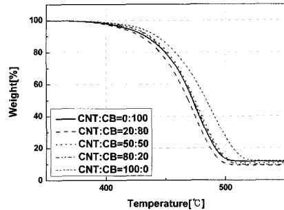
(a) CNT, CB 함량에 따른 TGA curve
