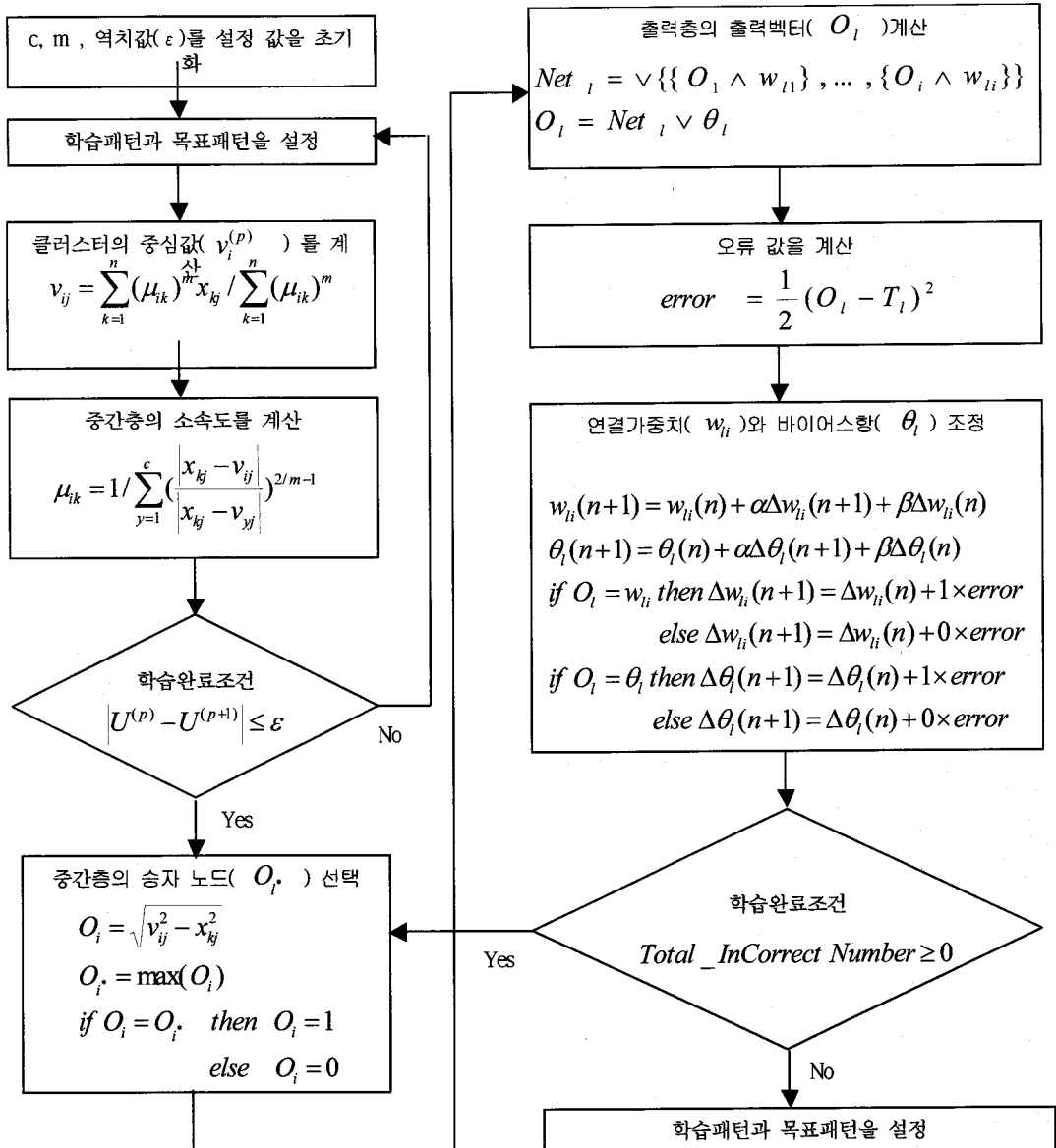
그림 7. 제안된 퍼지 신경망 Fig 7. The proposed fuzzy neural networks
