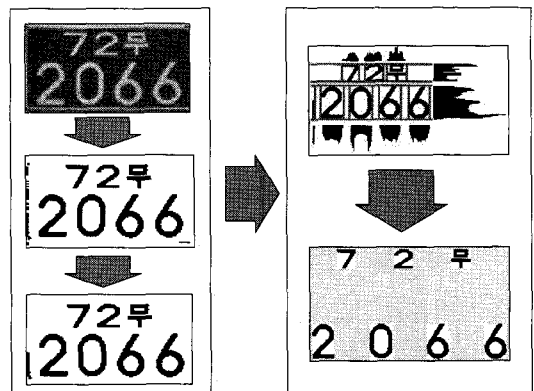
그림 6. 개별 코드 추출 Fig 6 Extraction of individual codes of vehicle number
