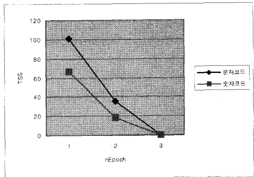
그림 12. 반복횟수에 따른 TSS 변화 과정 Fig 12. Change stage of TSS by epoch number
