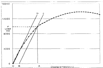
그림8. 장 플레이트의 골곡곡선 Fig.8 Schematized diagram of the Bending curve of Long plate
