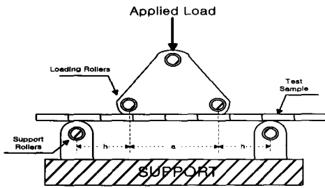
그림2. 뼈금속판의 굴곡구조 강성
