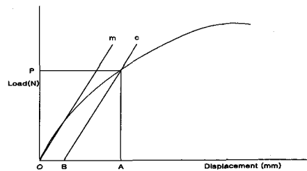
그림1. 금속판 굴곡곡선
