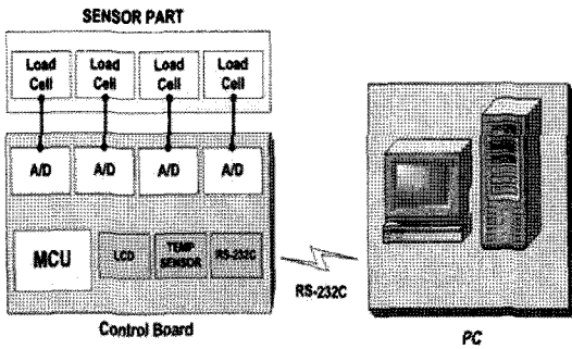
그림 1. 전체시스템의 구성도 Fig. 1. Schematics of the system.
