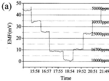
그림 4. 1000\text{ }^\circ\text{C} 에서 열처리된 Pd 전극을 NO_x 분해촉매로 사용하는 NO_x 센서의 700\text{ }^\circ\text{C} , 유량 300\text{ cc/min} 에서의 NO 감지 특성 (a) NO 농도에 따른 기전력변화, (b) 센서의 NO 에 대한 감도 그래프
