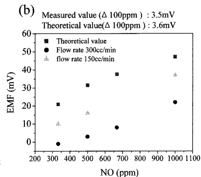
그림 5. 1300\text{ }^\circ\text{C} 에서 열처리된 Pd 전극을 NO_x 분해촉매로 사용하는 NO_x 센서의 700\text{ }^\circ\text{C} 에서의 NO 감지특성 (a) NO 농도에 따른 기전력변화, (b) 센서의 NO 에 대한 감도 그래프
