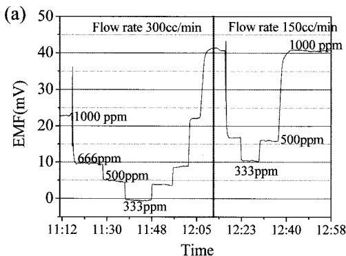
그림 5. 1300\text{ }^\circ\text{C} 에서 열처리된 Pd 전극을 NO_x 분해촉매로 사용하는 NO_x 센서의 700\text{ }^\circ\text{C} 에서의 NO 감지특성 (a) NO 농도에 따른 기전력변화, (b) 센서의 NO 에 대한 감도 그래프
