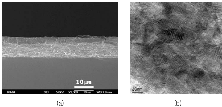
그림 22. Ti 기판위에 에어로졸 데포지션 공정으로 코팅한 hydroxyapatite: (a) 두께가 균일한 코팅층을 나타내는 SEM 사진, (b) 수십 나노미터 크기의 hydroxyapatite 결정립과 비정질로 구성된 치밀한 미세조직의 코팅을 보이는 HR-TEM 사진.
