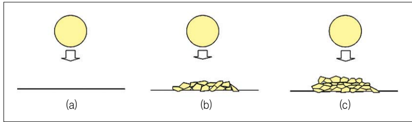
그림 2. 에어로졸 데포지션 코팅 과정; (a) 분사된 입자가 기판에 충돌함, (b) 입자가 분쇄되면서 일부 조각들이 기판에 박히거나 강력한 결합을 하고 다음 입자가 그 위에 충돌함, (c) 충돌된 입자가 분쇄되어 강한 결합을 이루는 층을 형성하고 다음 입자가 그 위에 충돌함.
