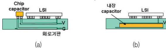
그림 13. 기판에 수동소자인 capacitor 실장 개략도; (a) 기존 기술인 표면 실장, (b) embedded capacitor [11] .
