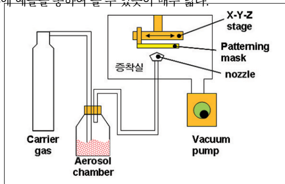
그림 1. 에어로졸 데포지션을 위한 장치의 개략도: 캐리어 가스가 세라믹 분말이 담긴 에어로졸 챔버로 유입되고 에어로졸 챔버 내에 부유하는 미세한 세라믹 분말들을 실어서 진공상태의 증착실 내에 있는 기판으로 노즐을 통하여 분사됨. 기판은 X축과 Y축으로 움직임.
