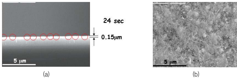
그림 3. 평균입경 0.8 마이크로미터의 분말을 사용한 PZT 세라믹 코팅층 (코팅시간 24초); (a) 단면 SEM사진, (b) 표면 SEM 사진.
