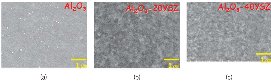
그림 18. 에어로졸 데포지션 공정으로 제작된 구조 기능 세라믹스 코팅: (a) 알루미늄, (b) 알루미늄-20wt% YSZ, (c) 알루미늄-40wt% YSZ; YSZ-Yttria Stabilized Zirconia.
