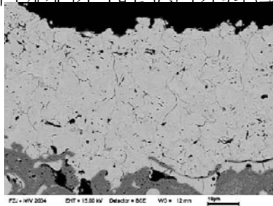
그림 5. 상압 플라즈마 용사공정으로 제작된 YSZ 코팅층의 단면 사진 [4] .
