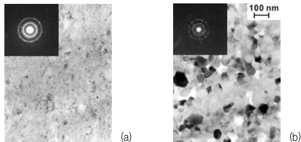
그림 16. 에어로졸 데포지션으로 제작된 NiZnCu ferrite 코팅층의 투과 전자 현미경 사진; (a) 코팅 직후, (b) 800 ^{\circ} C 공기 중에 5분간 열처리 후 [13] .
