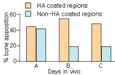
그림 21. 사체로부터 채취한 Ti계 인공 보철물의 표면에 뼈 조직이 덮힌 정도의 비교; 동일한 인공 보철물의 hydroxyapatite (HA) 코팅이 남아있는 부분과 벗겨진 부분에서의 뼈 세포 발달정도를 비교할 수 있음.
