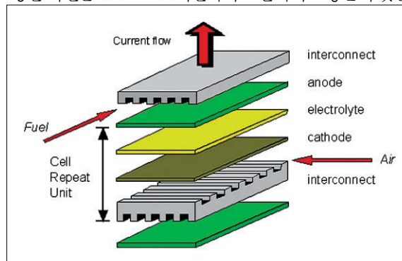
그림 20. SOFC stack의 기본 unit인 cell의 구조.
