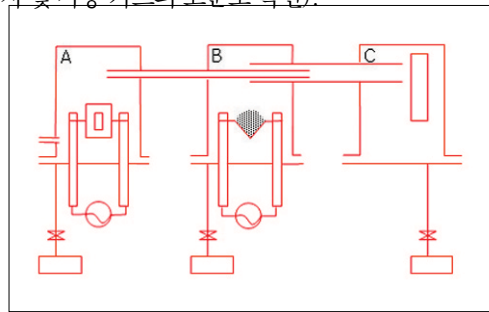
그림 7. Gas deposition 공정을 위한 장치의 주요부분 개략도; A, B-금속 원료 증발실, C-증착실; 금속 증발을 위한 발열체로 흑연 발열체, 몰리브덴 또는 텅스텐 발열체 사용 [7] .
