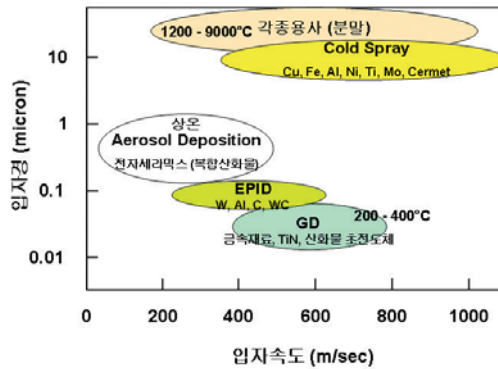
그림 8. 각종 분말 분사 코팅공정의 비교 [6] .
