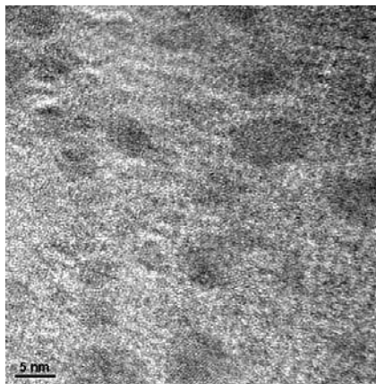
그림 4. 에어로졸 데포지션에 의해 제작된 PZT 코팅층의 고분해능 투과전자현미경 사진; 결정질을 나타내는 격자 이미지와 비정질을 확인할 수 있으며 결정질의 직경은 10nm 이하 임.
