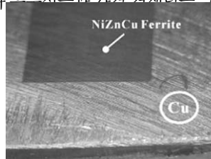
그림 15. 에어로졸 데포지션으로 제작된 NiZnCu ferrite의 사진 [13] .
