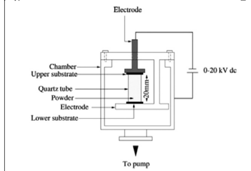
그림 6. EPID 공정을 위한 장치의 개략도 [5] .
