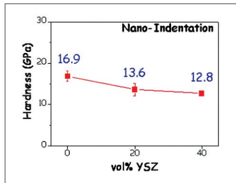
그림 19. YSZ의 함량에 따른 에어로졸 데포지션으로 제작된 알루미늄-YSZ 코팅층의 경도 변화 [14] .
