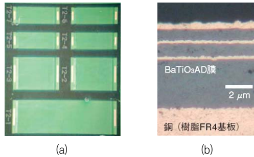
그림 14. Fujitsu사에서 개발한 에어로졸 데포지션에 의한 embedded capacitor용 BaTiO 3 유전체의 사진; (a) 표면, (b) 단면.
