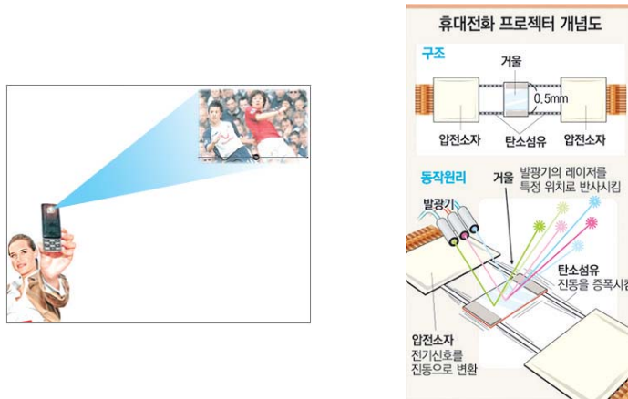
그림 12. 압전 mirror actuator를 채용한 휴대폰 프로젝션 디스플레이의 개념도 [10] .
