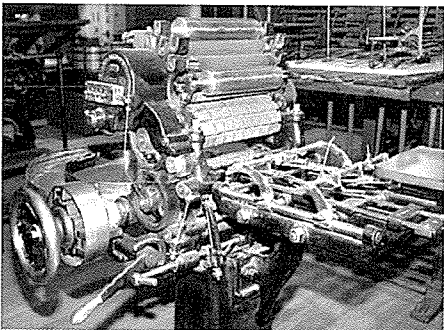
해리 E-1 자동엔버롭인쇄기
