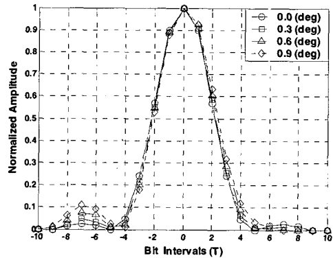
그림 5. 35GB BD 채널에서의 채널 임펄스 응답
