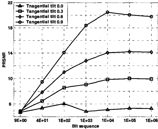
(b) 실제 채널의 tilt = 0.9° 그림 6. 비선형 채널에서 각 등화기의 PRSNR 값의 변화
