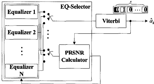
그림 7. PRSNR을 이용한 PRML 검출기
