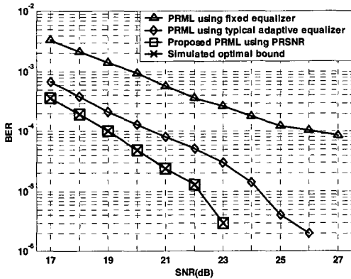
그림 9. Tilt 0.9°에서 제안한 PRML 검출방법과 일반적인 PRML 검출 방법의 BER 성능 비교
