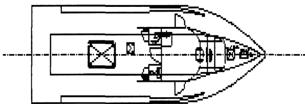
Fig. 26. Upper deck plan.
