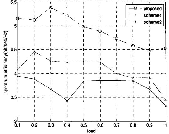
그림 7. load에 따른 채널당 전송률
