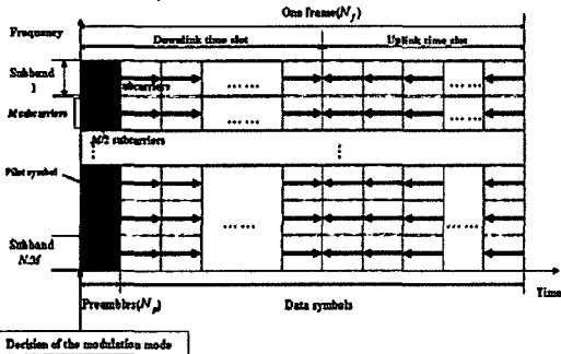
그림 2. 단일 사용자 부대역 프레임 크기
