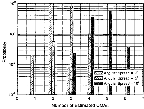
그림 10. 여러 angular spread에 대한 추정된 도래각 수의 분포
