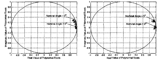
(a) 주파수 비 선택성 환경 (b) 지연 시간 = (0, 7 \mu s, 10 \mu s) 그림 7. 지연 확산에 따른 root-MUSIC 알고리즘의 성능.
