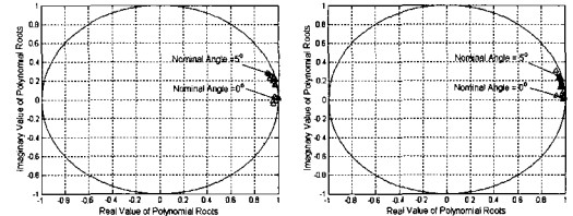
(a) 부 반송파 = 256, OFDM 심볼 = 1 (b) 부 반송파 = 32, OFDM 심볼 = 8 그림 8. 부 반송파와 OFDM 심볼 수에 따른 root-MUSIC 알고리즘의 성능.
