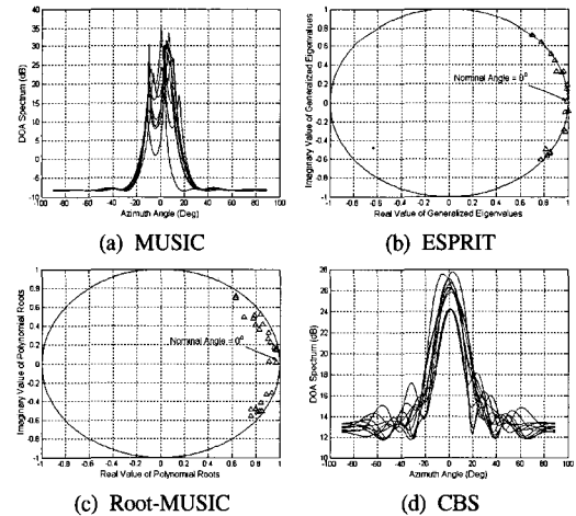
그림 9. Angular spread 발생 시 초 분해능 방향 탐지 알고리즘과 CBS 알고리즘의 성능 비교
