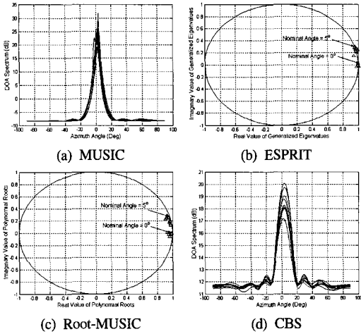
그림 6. 초 분해능 방향 탐지 알고리즘과 CBS 알고리즘의 성능 비교(0°, 5°).
