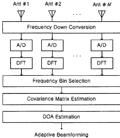
그림 3. OFDMA 스마트 안테나 시스템을 위한 초 분해능 방향 탐지 시스템의 구조
