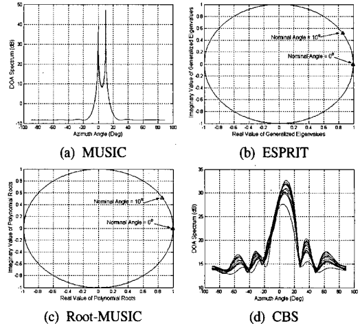
그림 5. 초 분해능 방향 탐지 알고리즘과 CBS 알고리즘의 성능 비교(0°, 10°).
