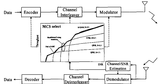
그림 1. 적응변조 및 부호화 시스템 구조(IV장: 표1. MCS레벨 참조)
