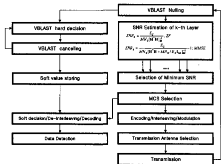
그림 4. AMC-V-BLAST 결합시스템 동작 구성도
