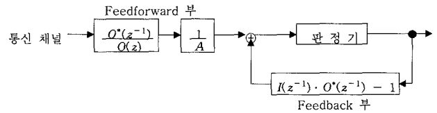
(그림 4) 결정 케환형 적응 등화기의 구조
