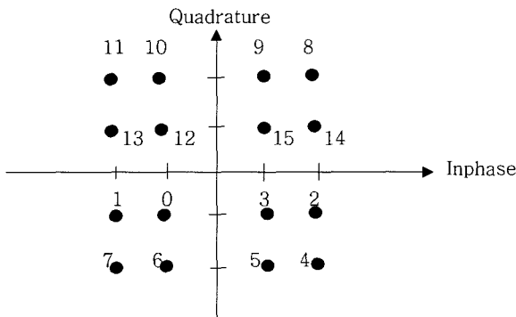
(그림 3) 사전 부호화후의 16-QAM 신호점 할당도
