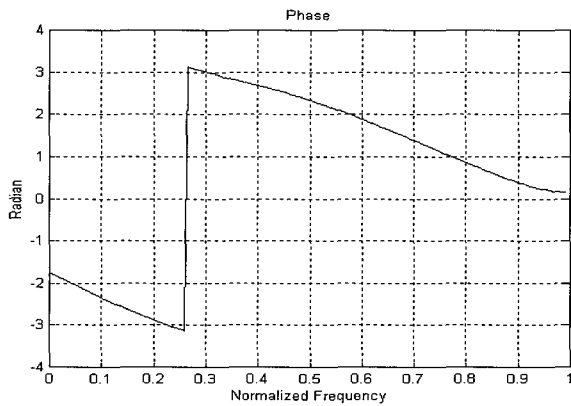
(b) 위상 특성
