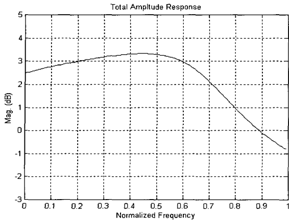
(a) 진폭 전달 특성
