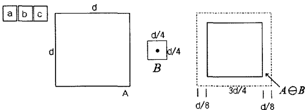
(그림 8) 침식연산
