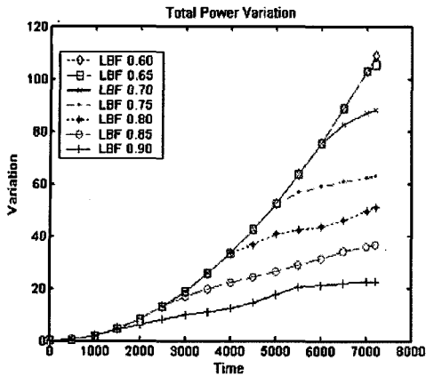
그림 7. LBF 값의 변화에 따른 노드 전력의 분산
