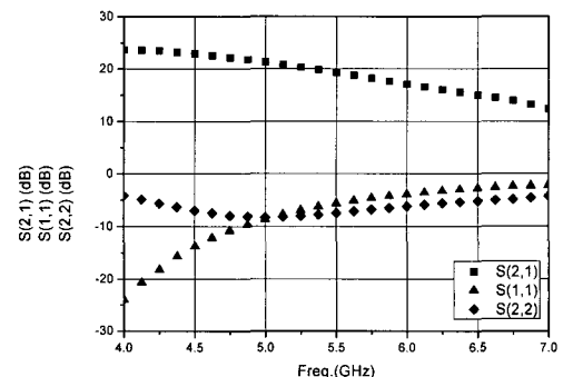
그림 6. 제작된 증폭기의 소신호 측정 결과
