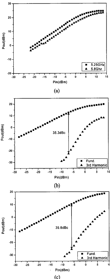
그림 7. 제작된 전력증폭기의 (a) 1-tone 측정, (b) 2-tone 측정을 통한 IMD3 (5.25GHz), (c) 2-tone 측정을 통한 IMD3 (5.8GHz)
