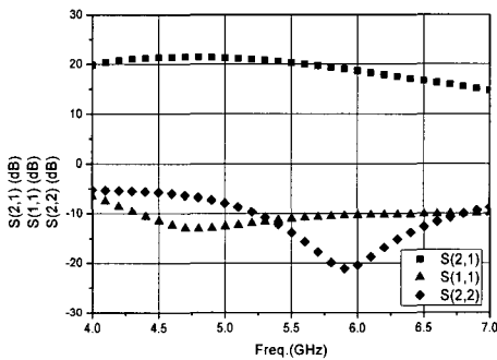
그림 4. 전력 증폭기의 소신호 주파수 특성, S21, S11, S22
