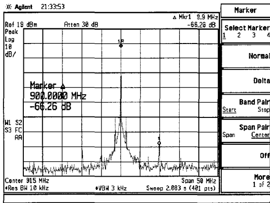
<Fig. 7> RF Module spectrum data
