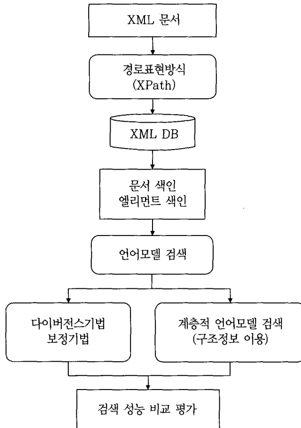
〈그림 2〉 XML 문서검색의 실험과정
