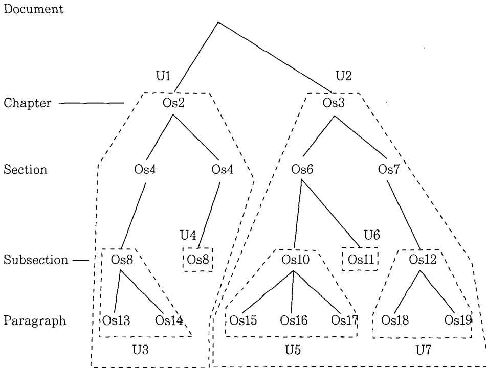
〈그림 1〉 FERMI 모델에서 규정한 문서의 구조 (Chiararella, Mulhem, and Foural 1996, 33)
